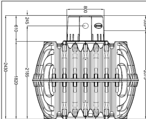
Depósito Carat con cubierta paso peatones
